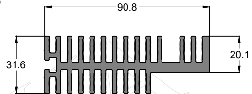
SEC.NO. IS0072 WEIGHT - 3.250 Kg/M
