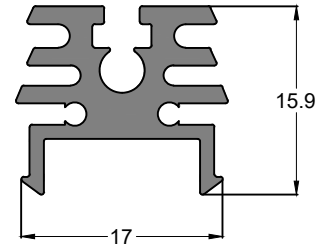
SEC.NO. IS0072 WEIGHT - 3.250 Kg/M
