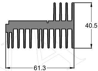
SEC.NO.IS00119 WEIGHT - 1.20 Kg/M
