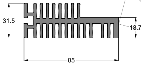
SEC.NO. IS0073 WEIGHT - 2.90 Kg/M
