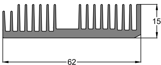
SEC.NO.IS0087 WEIGHT - 1.20 Kg/M
