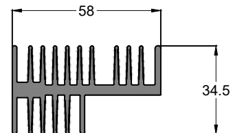
SEC.NO.IS0086 WEIGHT - 1.80 Kg/M
