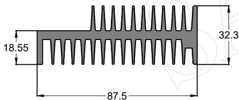
SEC.NO. IS0073 WEIGHT - 2.90 Kg/M
