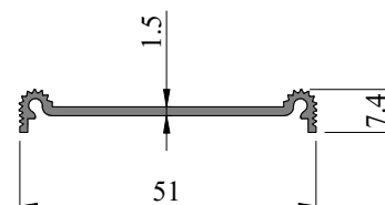
SEC.NO.IS0069 WEIGHT - 0.340 Kg/M
