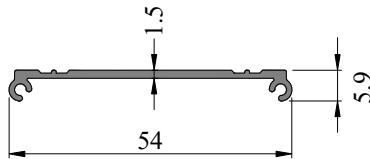
SEC.NO. IS0040 WEIGHT - 0.245 Kg/M
