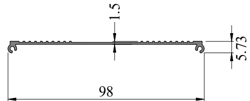
SEC.NO.IS0006 WEIGHT - 0.340 Kg/M
