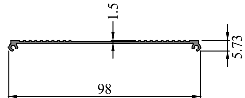
SEC.NO.IS0006 WEIGHT - 0.340 Kg/M
