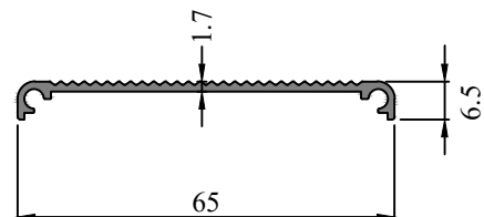
SEC.NO.IS0098 WEIGHT - 0.300 Kg/M
