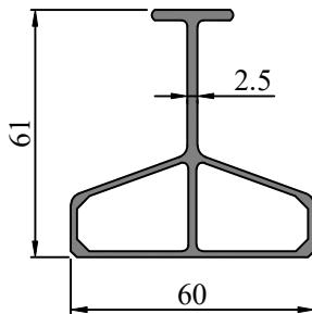
SEC.NO. IS0015 WEIGHT - 1.20 Kg/M
