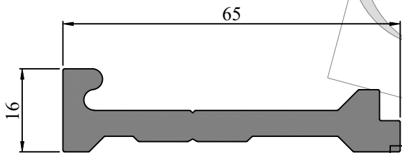
SEC.NO. IS0015 WEIGHT - 1.20 Kg/M
