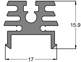
SEC.NO. IS0072 WEIGHT - 3.250 Kg/M
