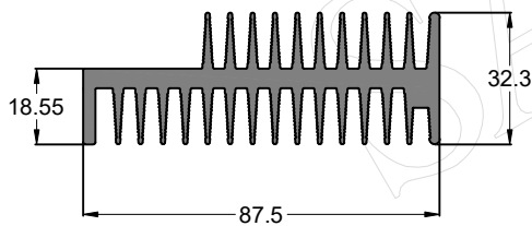
SEC.NO. IS0073 WEIGHT - 2.90 Kg/M
