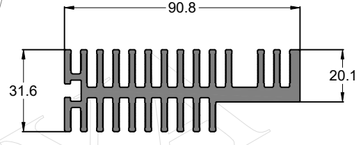
SEC.NO.IS0086 WEIGHT - 1.80 Kg/M
